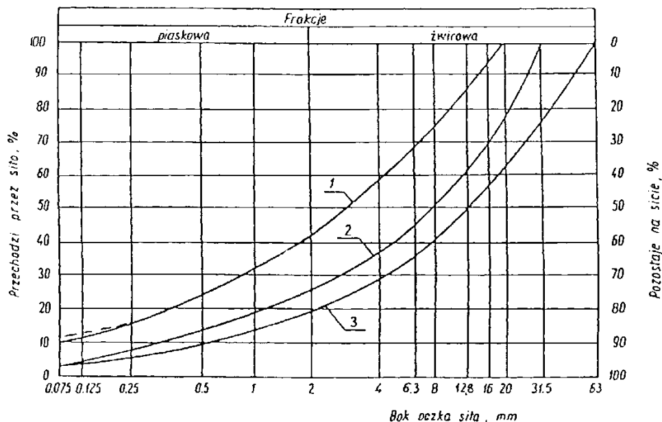
Rysunek 1. Pole dobrego uziarnienia kruszyw przeznaczonych na nawierzchnię wykonywaną metodą stabilizacji mechanicznej
